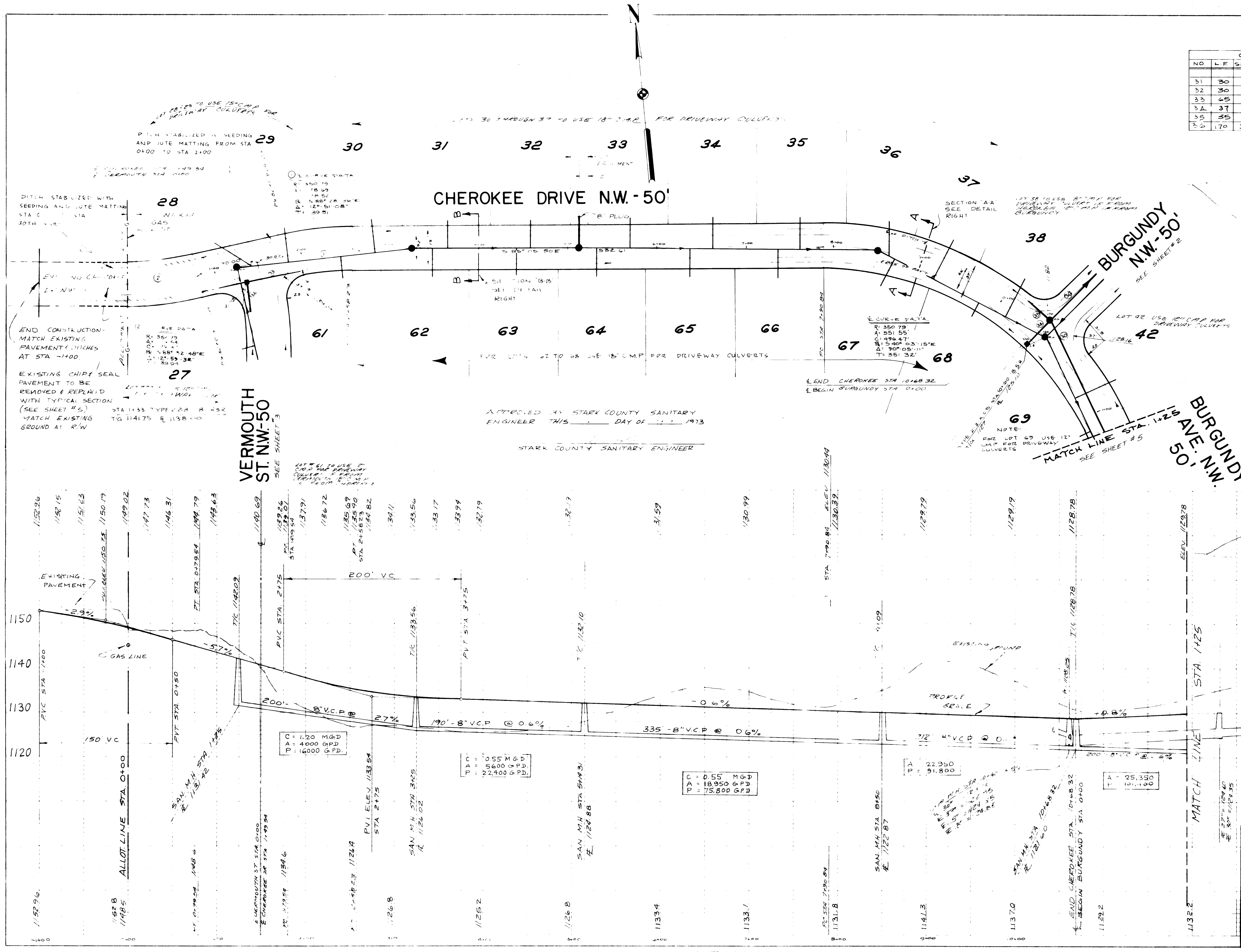
SECTION "A-A" SCALE: 1"=20' HORIZ., 1"=10' VERT.
