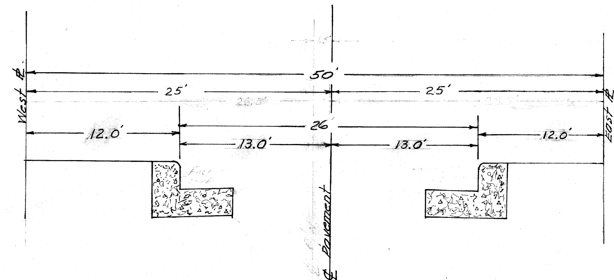
SECTION A-A
