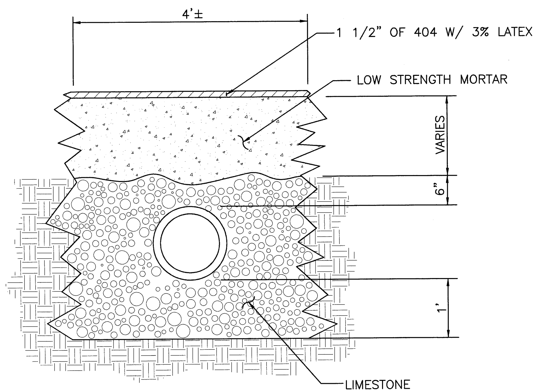
SECTION C-C SCALE: 1=1
