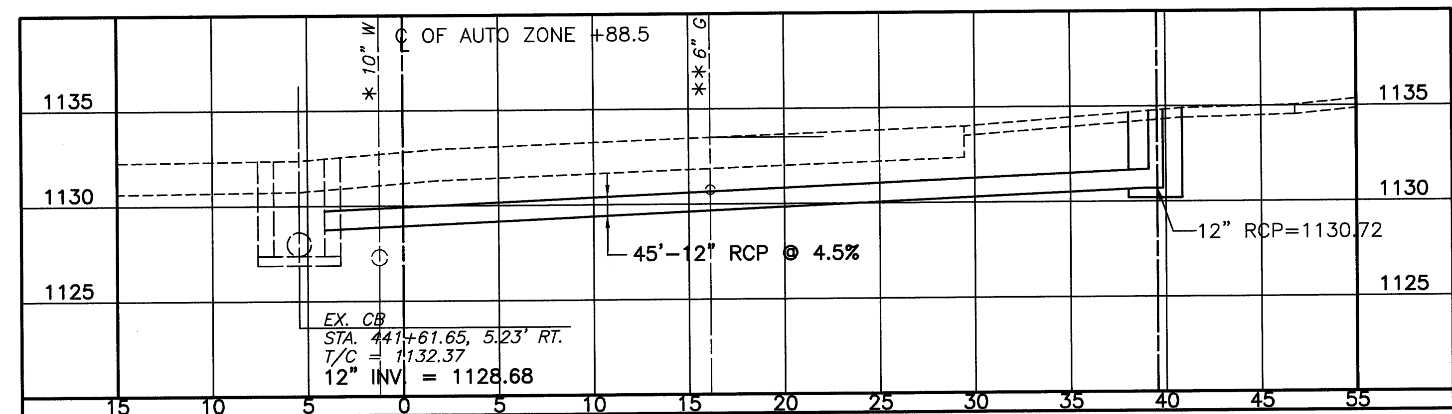
SECTION B-B SCALE: 1=5
