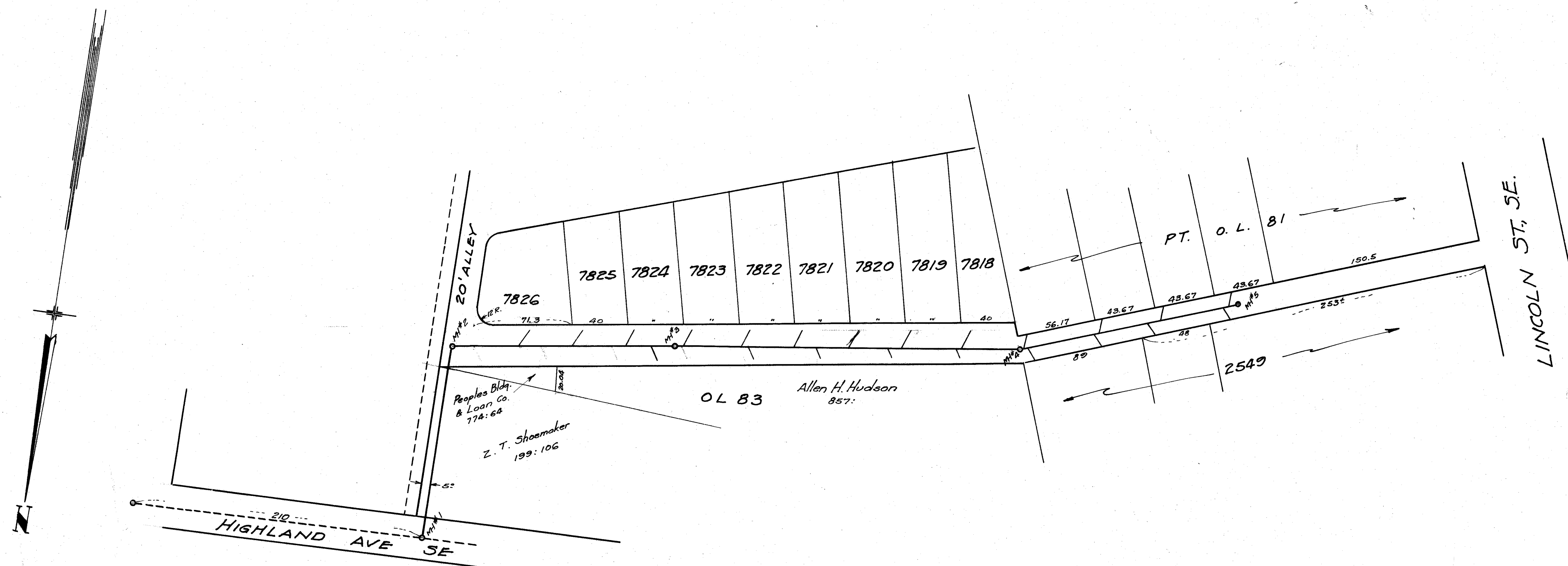
DIELHENN AVE, SE, SAN. SEWER
