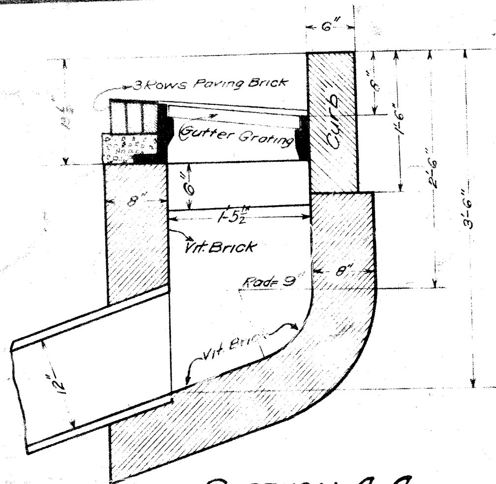
SECTION A-A
