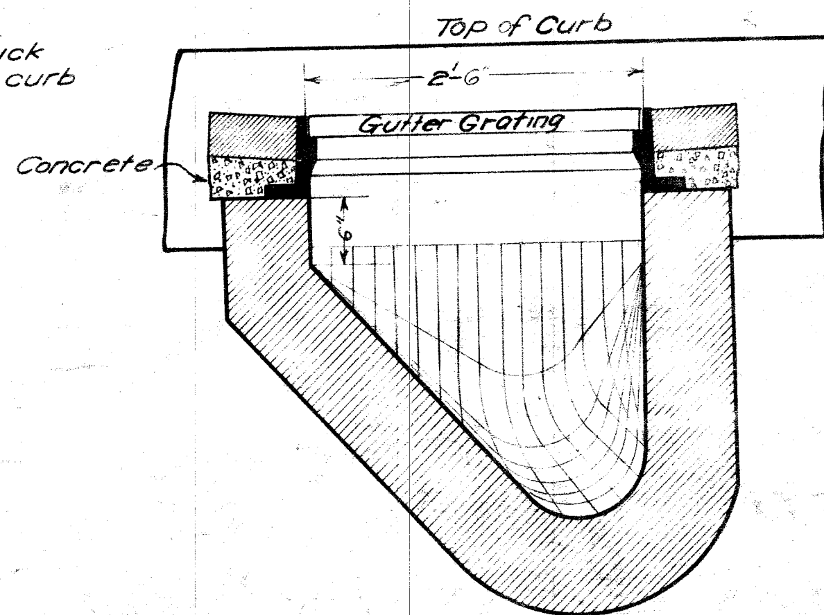
ELEVATION B-B
