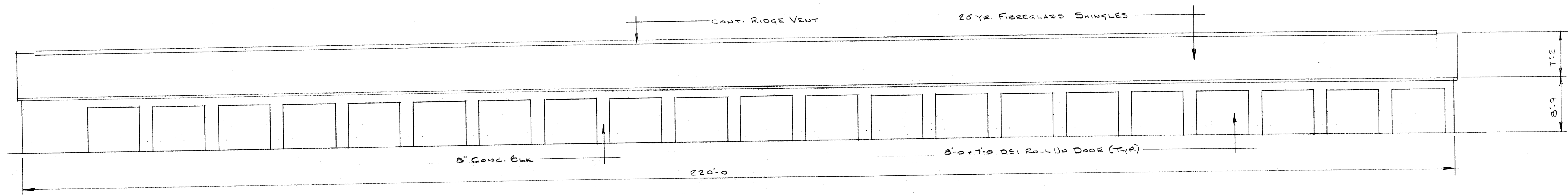
WEST ELEVATION SCALE: \frac{1}{8}'' = 1'-0''
