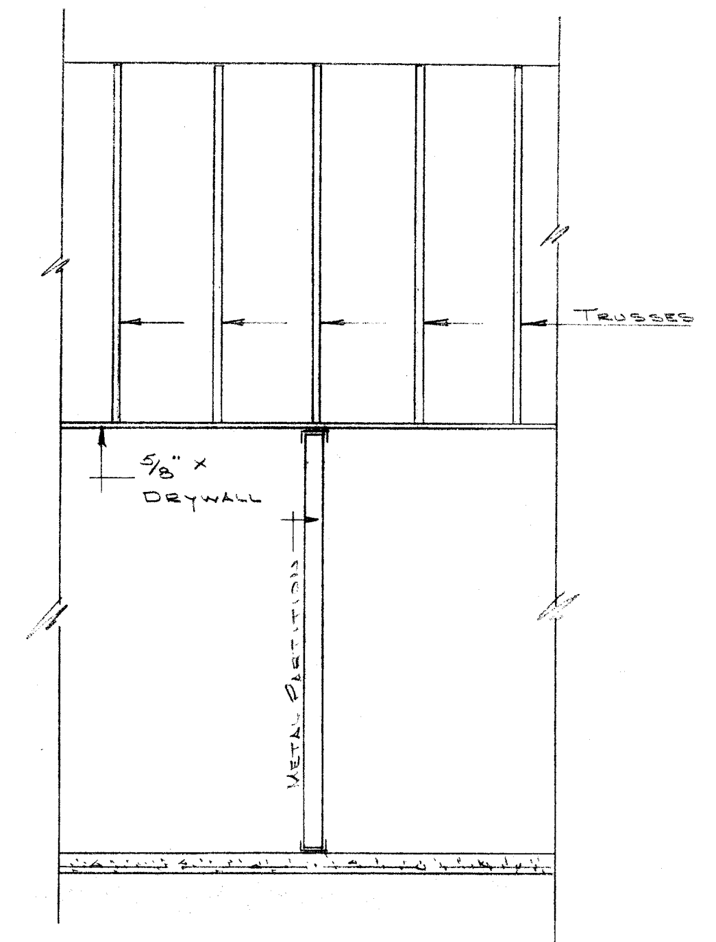
SECTION B-B (SHEET A-1) SCALE: 3/8" = 1'-0"
