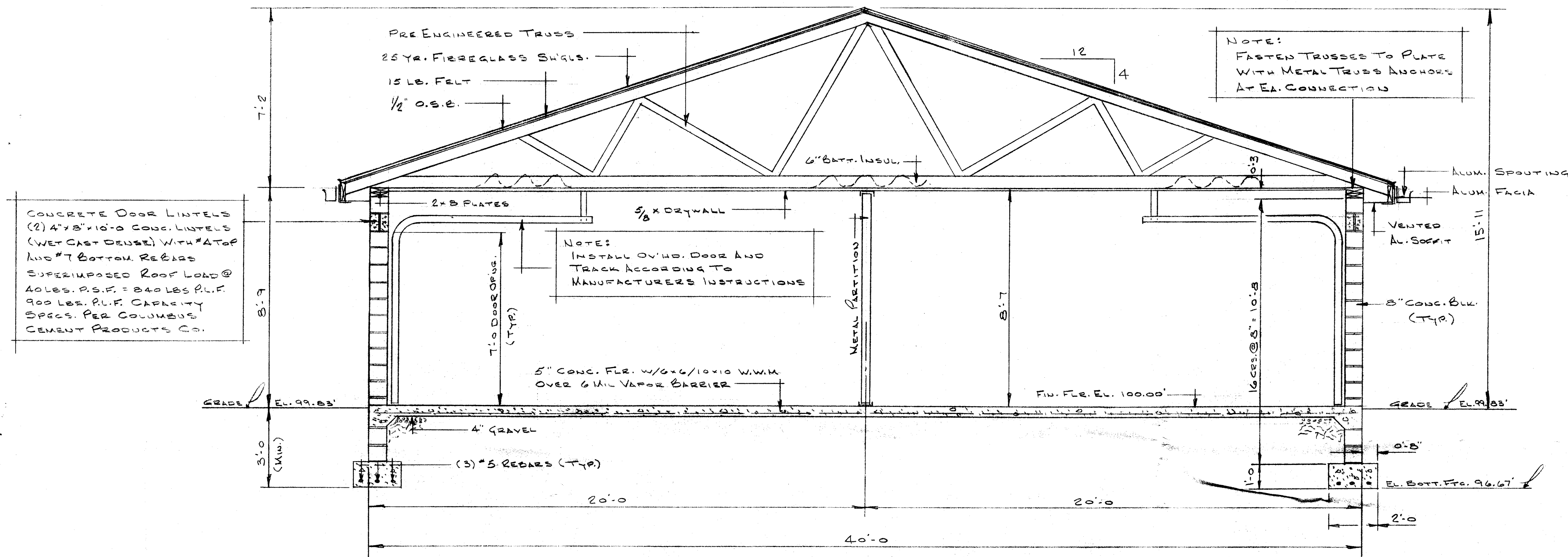
SECTION A-A (SHEET A-1) SCALE: 3/8" = 1'-0"
