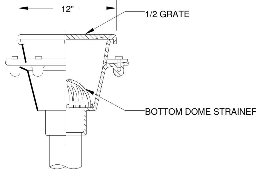
FLOOR SINK DETAIL N.T.S.
