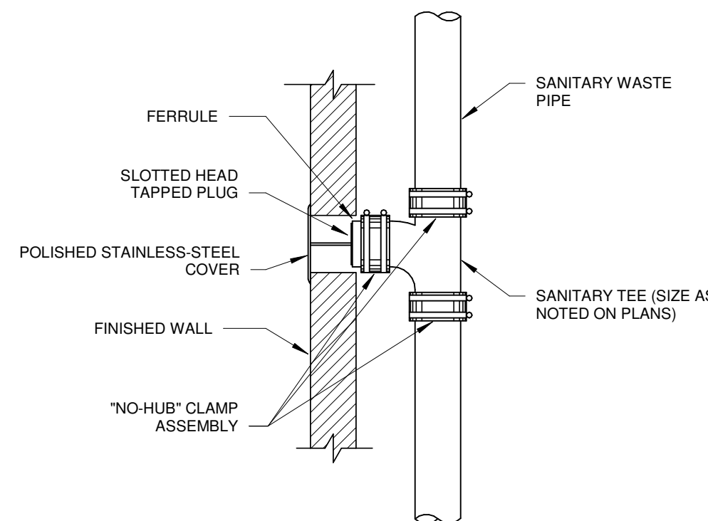
WALL CLEANOUT DETAIL N.T.S.
