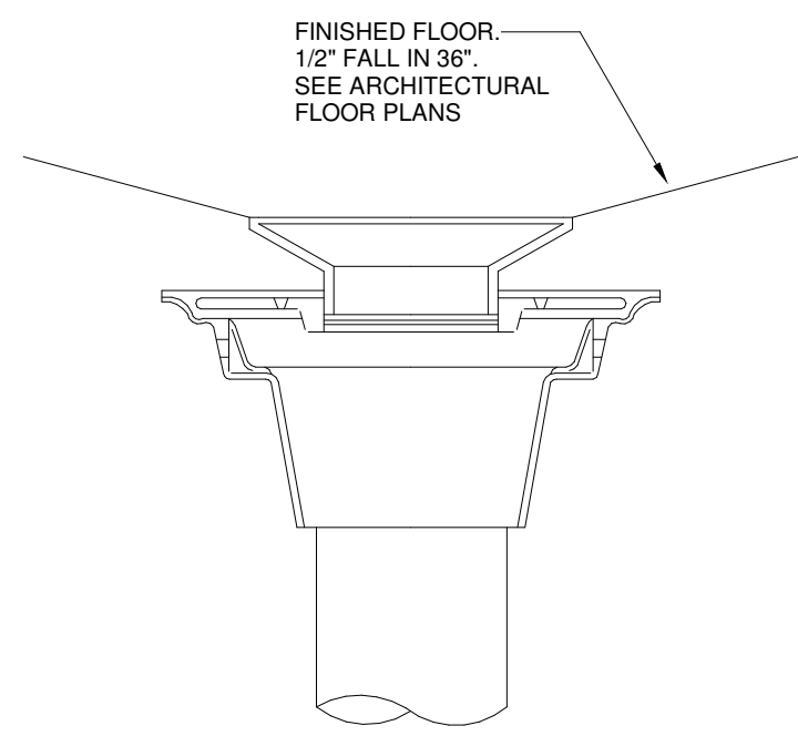
FLOOR DRAIN DETAIL N.T.S.
