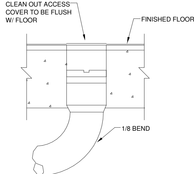
FLOOR CLEANOUT DETAIL N.T.S.
