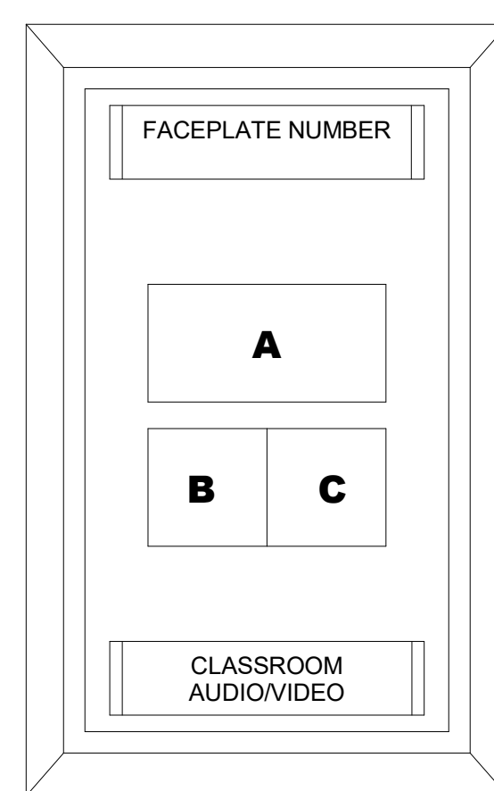
TYPE "AV" FACEPLATE DETAIL SCALE: NONE
