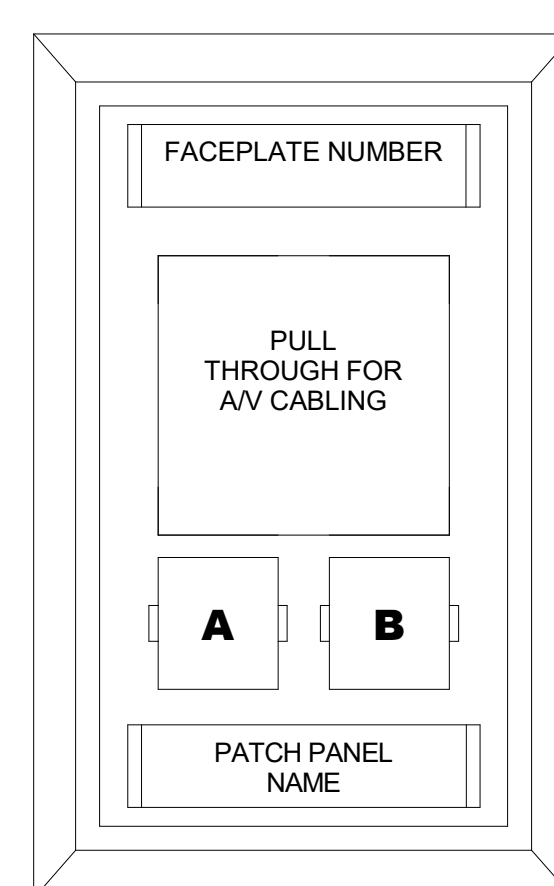
TYPE "VM" FACEPLATE DETAIL SCALE: NONE
