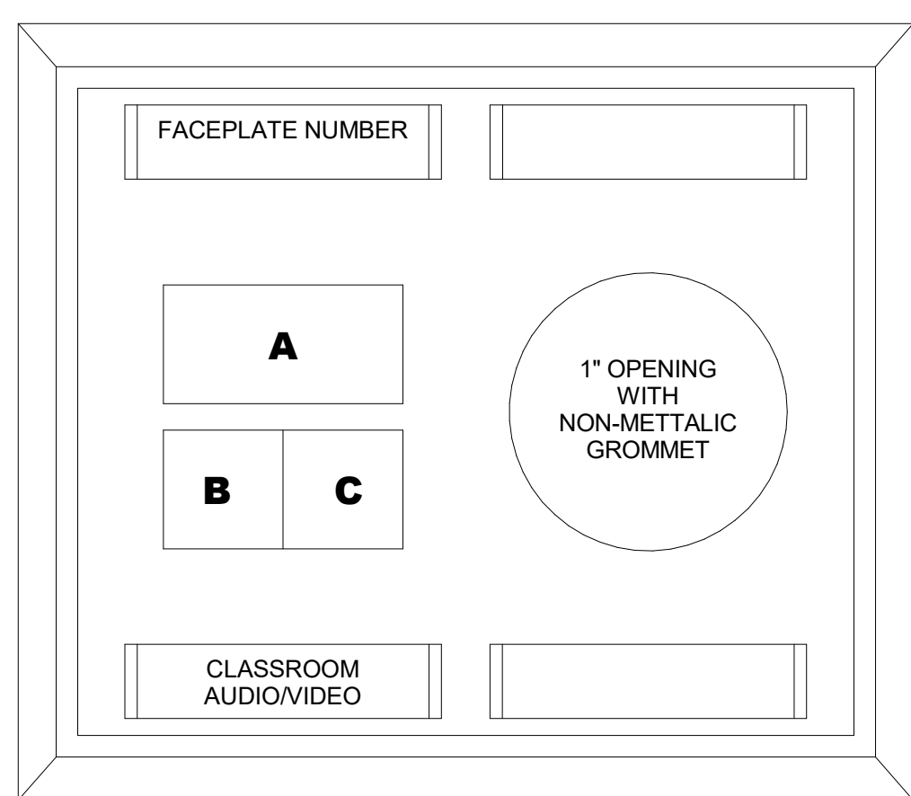
TYPE " AV " FACEPLATE DETAIL SCALE: NONE
