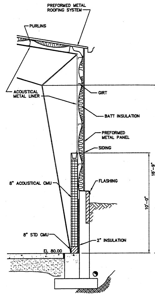
SECTION D SCALE: 3/8"=1'-0" A9,10,11
