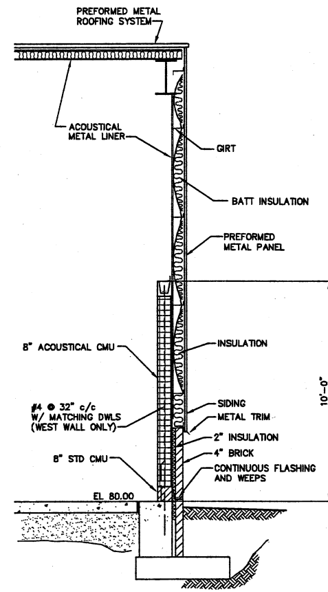
SECTION C SCALE: 3/8"=1'-0" A9,10,11
