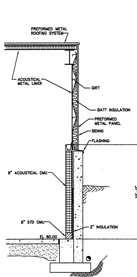
SECTION E SCALE: 3/8"=1'-0" A9,10,11
