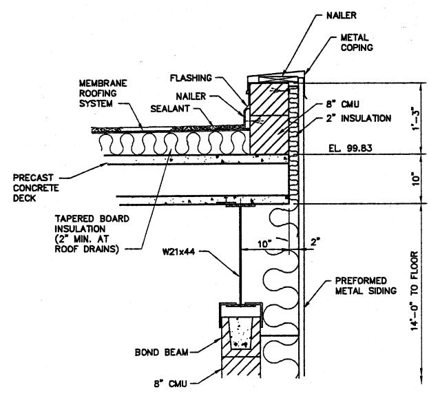
SECTION 1 SCALE: 1"=1'-0"
