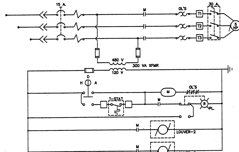
EXHAUST FAN EF-2 (BLOWER BUILDING)
