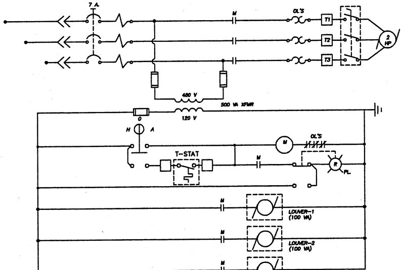
EXHAUST FAN EF-2 (BLOWER BUILDING)
