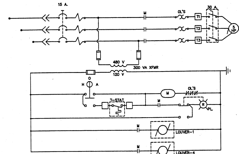
EXHAUST FAN EF-3 (BLOWER BUILDING)
