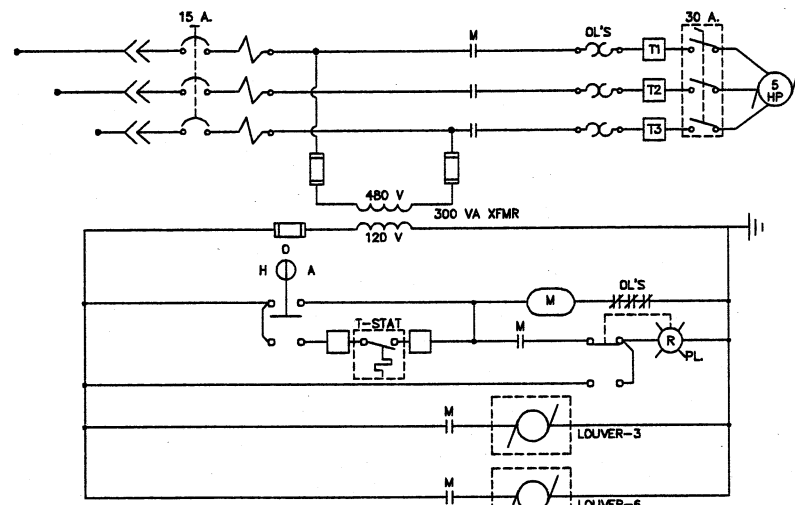
EXHAUST FAN EF-1 (BLOWER BUILDING)
