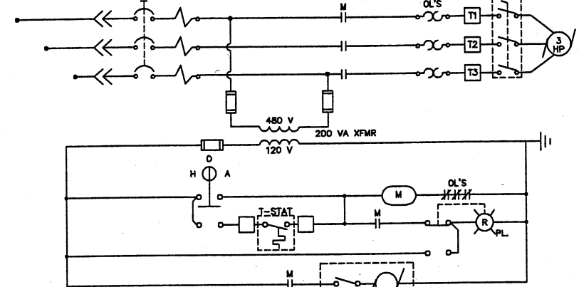
EXHAUST FAN EF-3 (BLOWER BUILDING)
