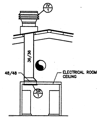
SECTION SCALE: 1/8"=1'-0" B M9
