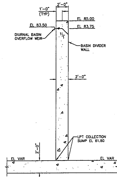
SECTION SCALE: 1/4\"/>
