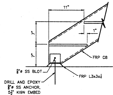
DETAIL 1 SCALE: 1 1/2" = 1'-0"
