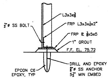
DETAIL 3 SCALE: 1 1/2" = 1'-0"
