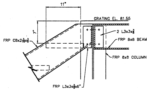
DETAIL 2 SCALE: 1 1/2" = 1'-0"
