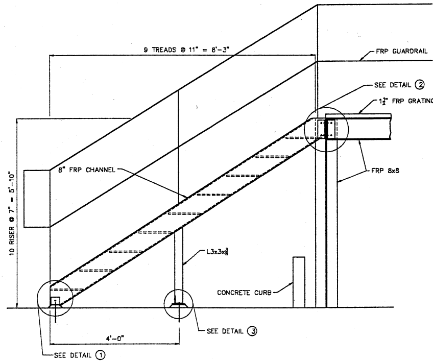
SECTION B SCALE: 3/4" = 1'-0"
