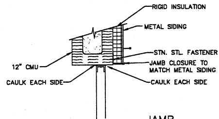
JAMB
