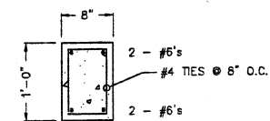
SECTION SCALE: 1" = 1'-0" (E)
