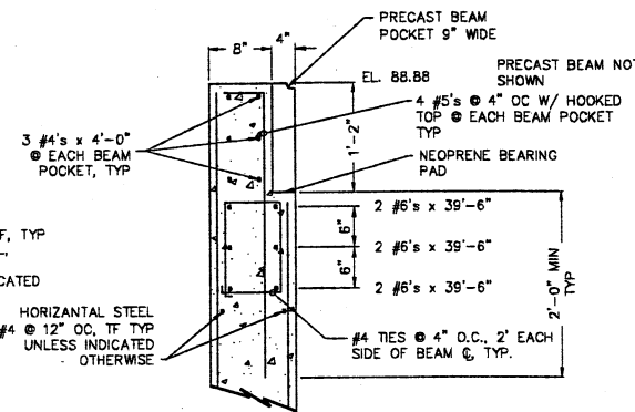
BEAM POCKET SECTION (D) SCALE: 1" = 1'-0"
